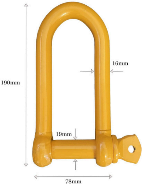
スチール製 使用荷重2000Kg
