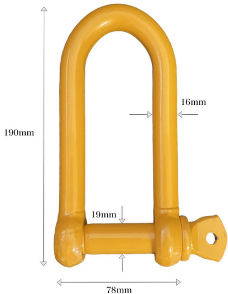
スチール製 使用荷重2000Kg
